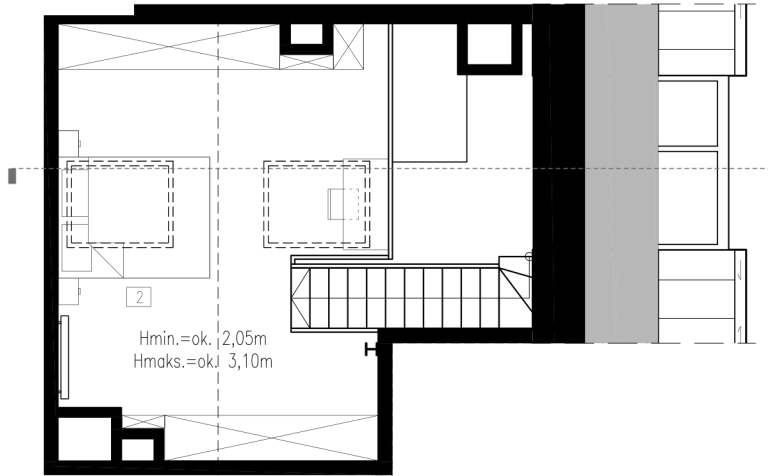
POZIOM + I
