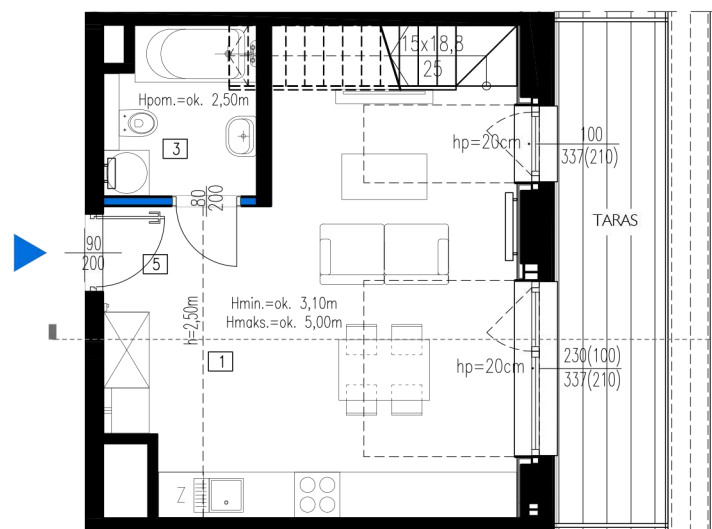
POZIOM 0
