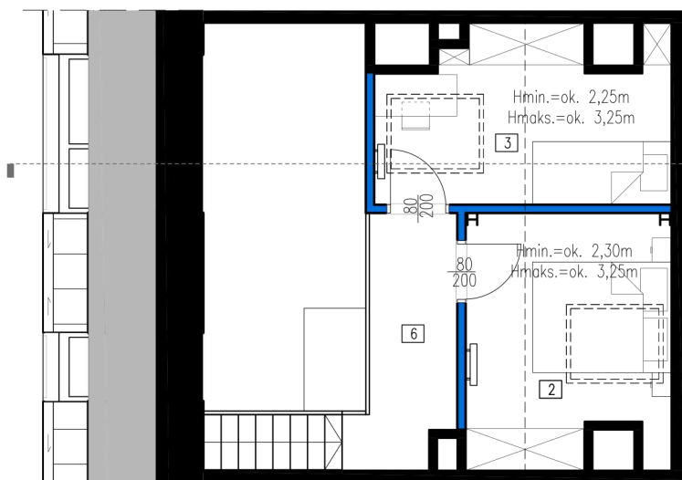
POZIOM + I
