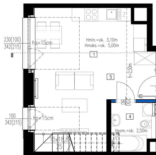
POZIOM 0
